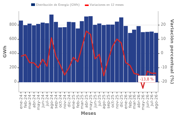
■ Evolución Distribución de Energía, región de Antofagasta (enero 2024 - agosto 2026)
