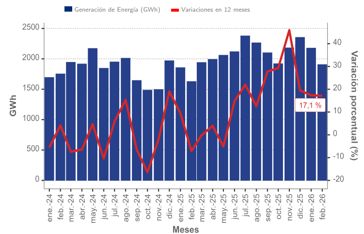
■ Evolución Generación de Energía, región de Antofagasta (enero 2024 - febrero 2026)
